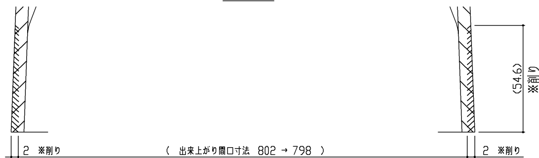
断面A-A
