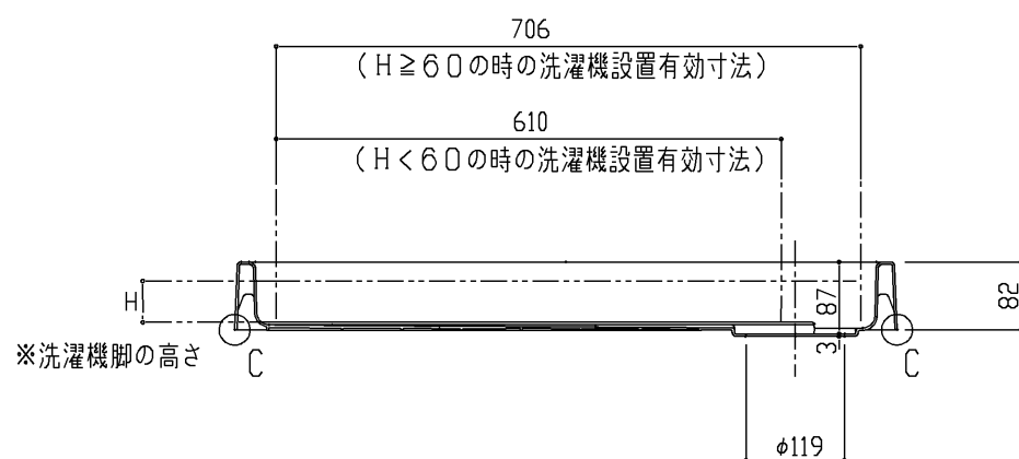
断面A-A
